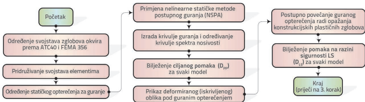
Slika 3. Drugi korak; procedura PBSD-a za dobivanje D_{pp} i D_{LS}
