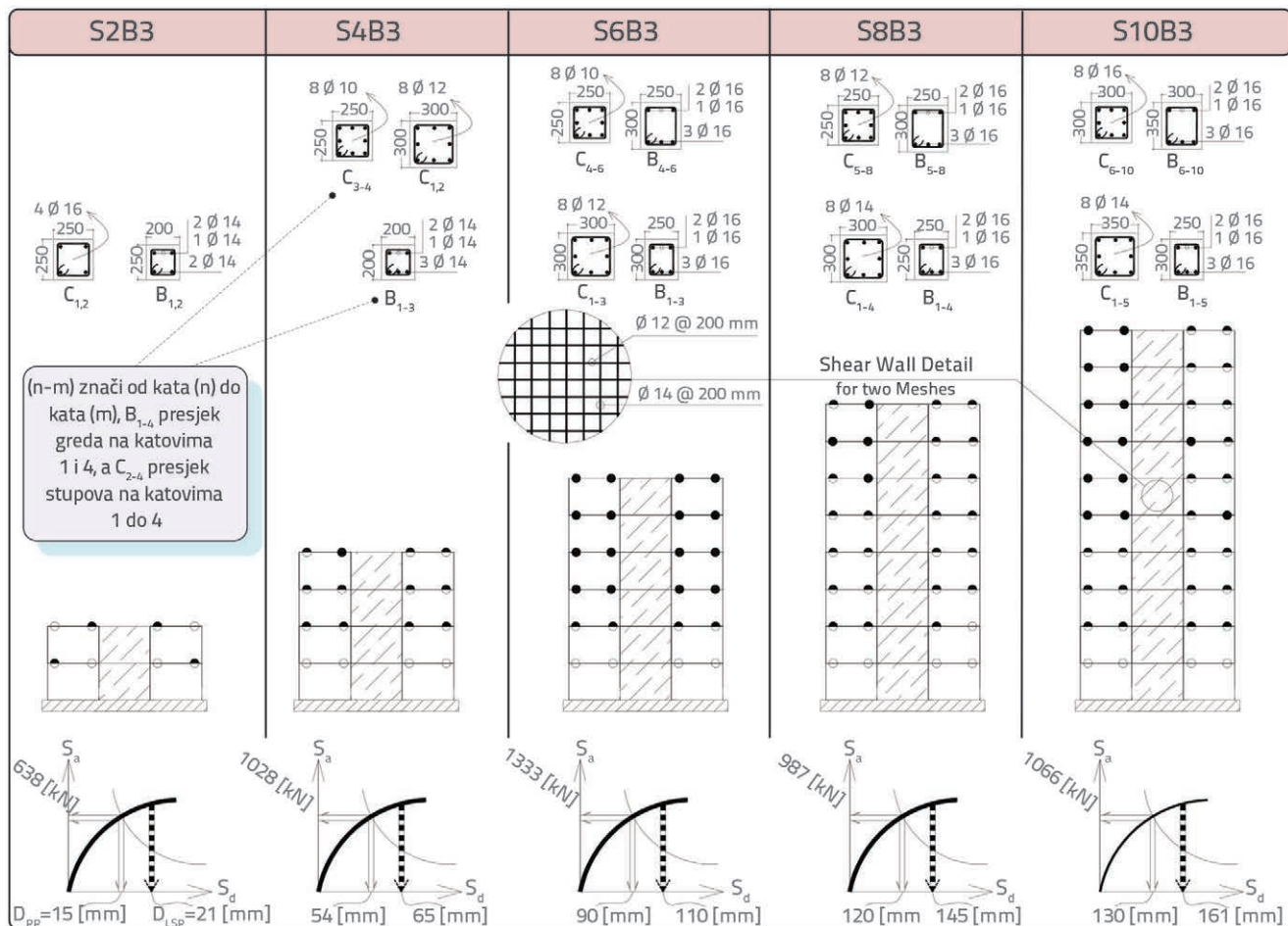
Slika 7. Svojstva presjeka stupova i gređa, mehanizam nastanka plastičnih zglobova propisanih svojstava i njihove shematske krivulje nosivosti u četvrtom koraku
