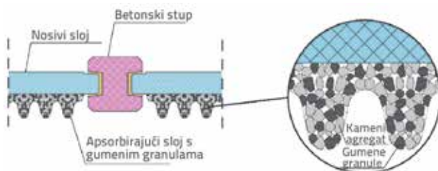
Slika 5. Poprečni presjek inovativnog rješenja RUCONBAR [28]
