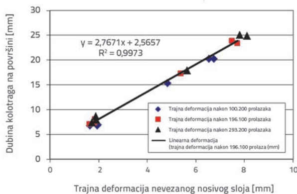
Slika 7. Korelacija između dubine kolotruga na površini i trajne deformacije nevezanog sloja šljunka debljine 15 cm na pokusnim konstrukcijama I i II
