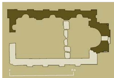
Tlocrt ostataka crkve Sv. Tome u Kutima pokraj Herceg Novog
