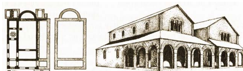
Tlocrt i rekonstrukcija dvojnih crkava u Mogorjelu pokraj Čapljine
