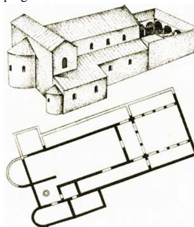
Rekonstrukcija i tlocrt crkve u Blagaju pokraj Bosanskog Novog
