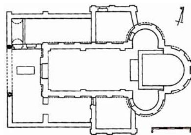
Tlocrt starokršćanske crkve na Dedića punti u Bilicama
